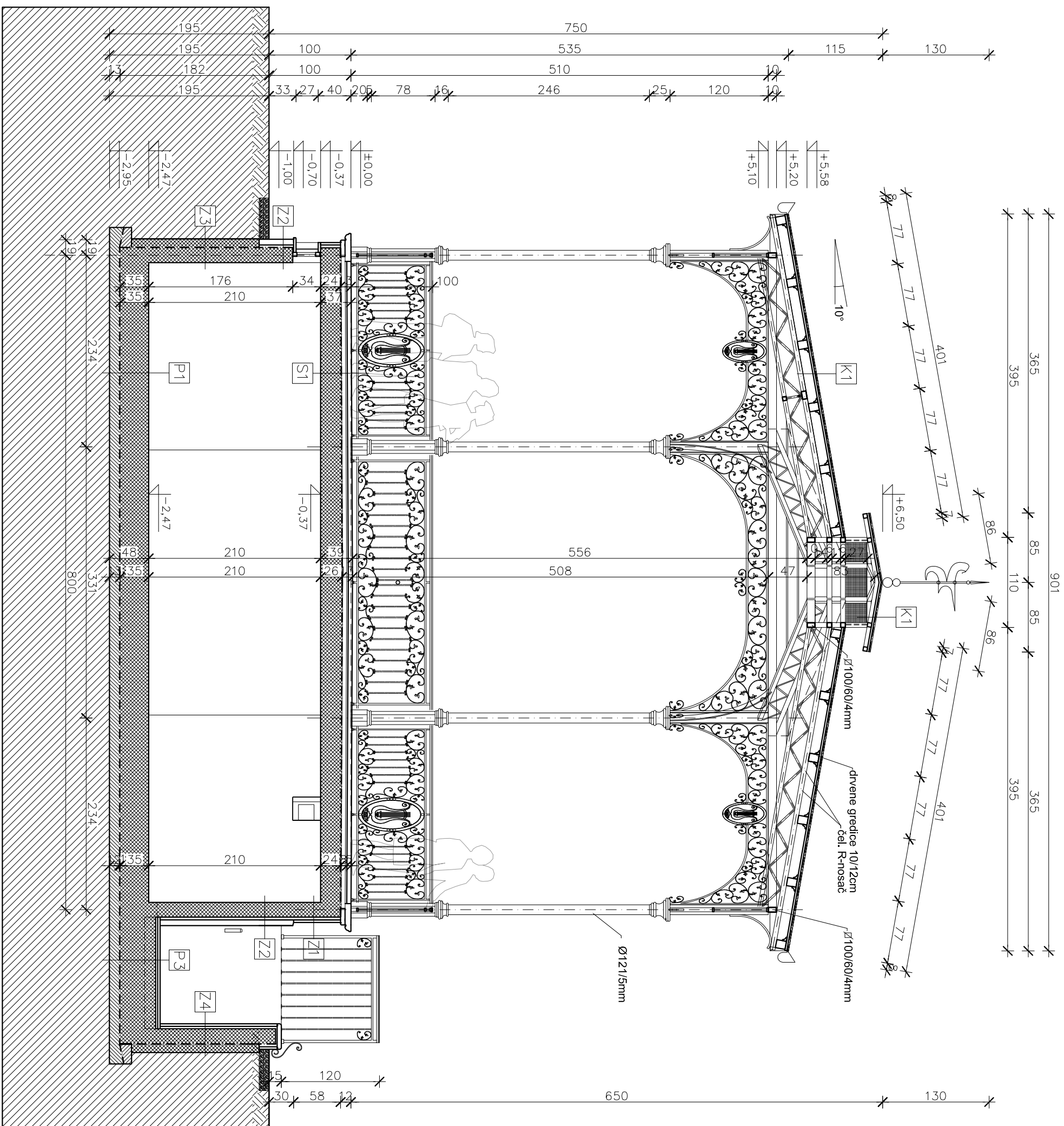
PRESJEK B-B 1:50
