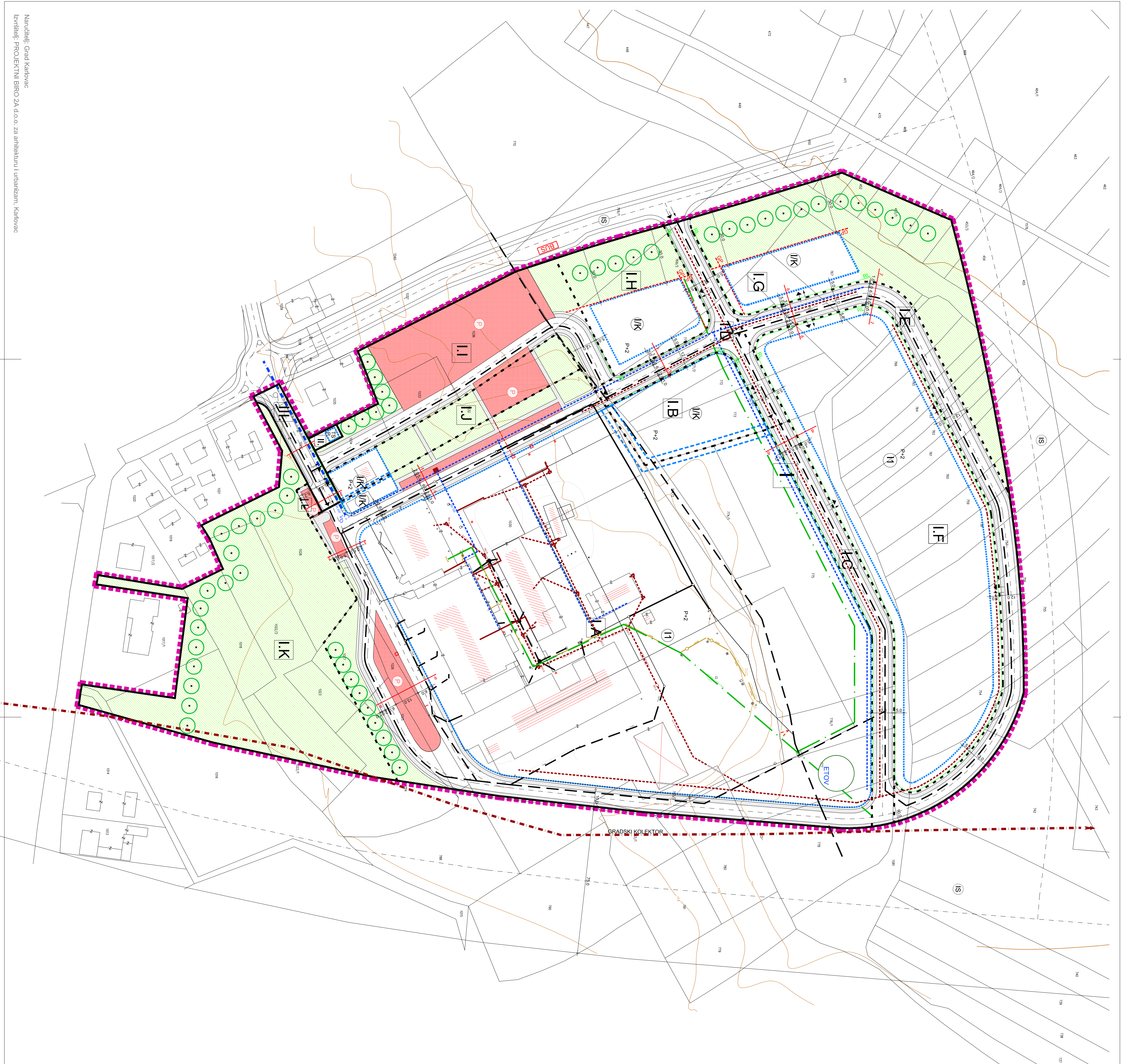
PROMET - PROFILU PROMETNICA
