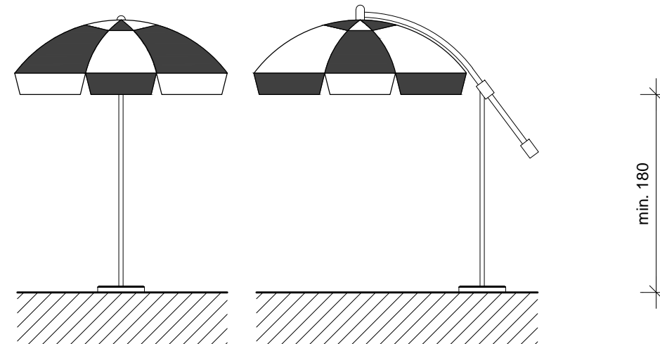
POGLED SUNCOBRANA
