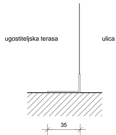
POGLED - PRIJEDLOG 07
