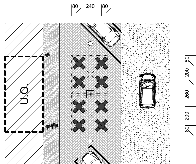
TLOCRT RASPOREDA NAMJEŠTAJA
