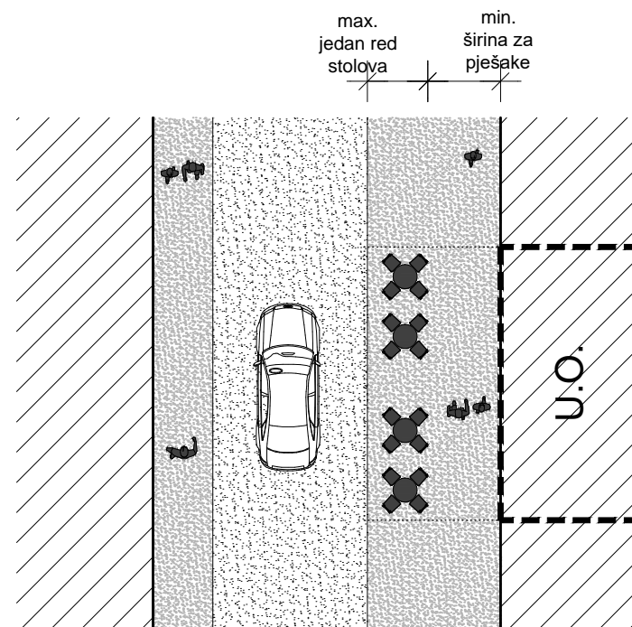
TLOCRT RASPOREDA NAMJEŠTAJA
