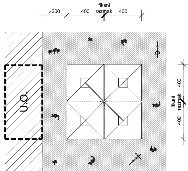
TLOCRT ČETVEROSTRUKOG SUNCOBRANA
