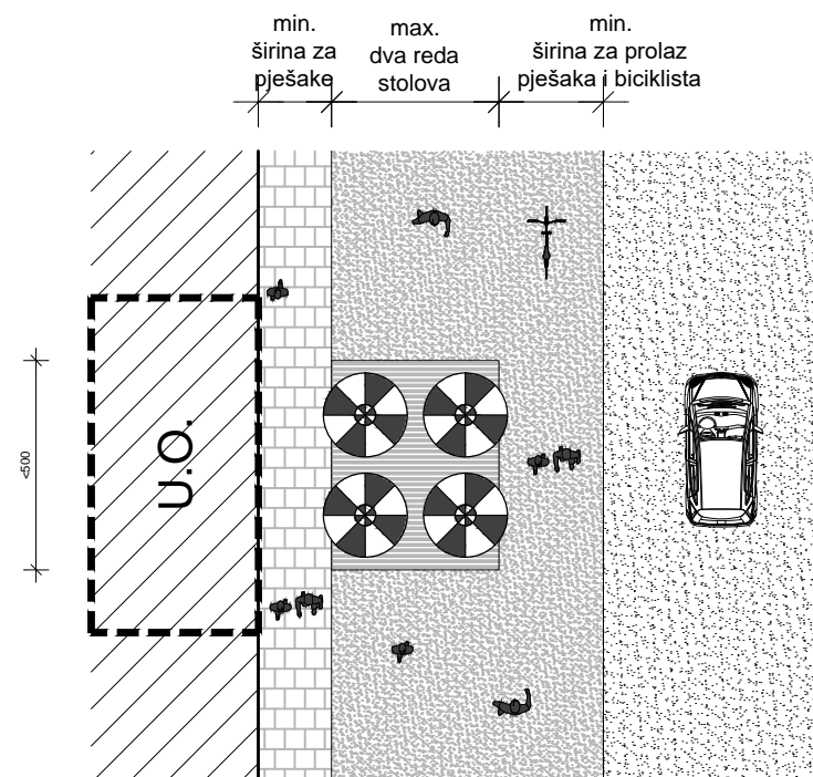
TLOCRT MALIH SOLITERNIH SUNCOBRANA
