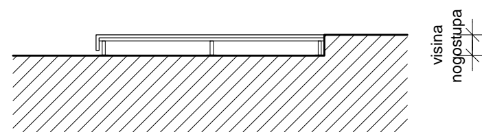
TLOCRT / POGLED PODIJA TERASE ZA IZJEDNAČAVANJE SA RAZINOM NOGOSTUPA
