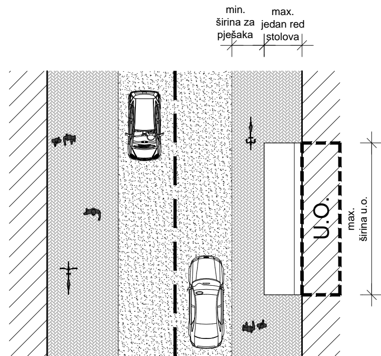
TLOCRT JEDNOSTREŠNIH TENDI
