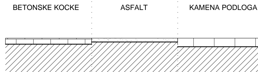
TLOCRT / PRESJEK BETONSKIH / ASFALJNIH / KAMNIH PLOHA
