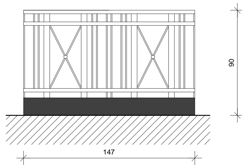
PRIJEDLOG 03 - KOVANO ŽELJEZO
