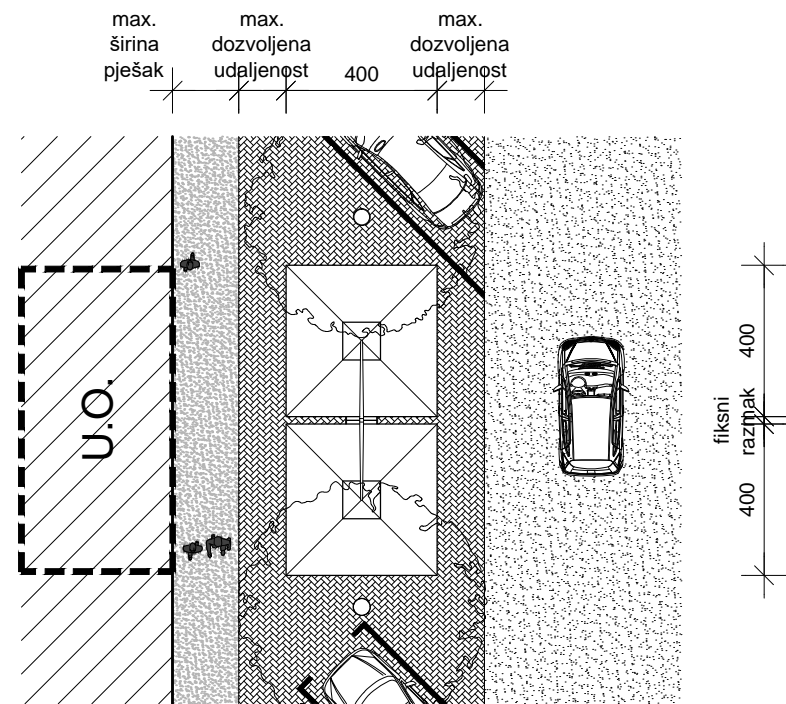
TLOCRT DVOSTRUKOG SUNCOBRANA
