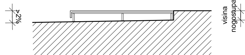
TLOCRT / POGLED PODIJA TERASE ZA IZJEDNAČAVANJE SA RAZINOM NOGOSTUPA
