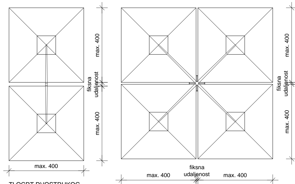
TLOCRT ČETVEROSTRUKOG SUNCOBRANA
