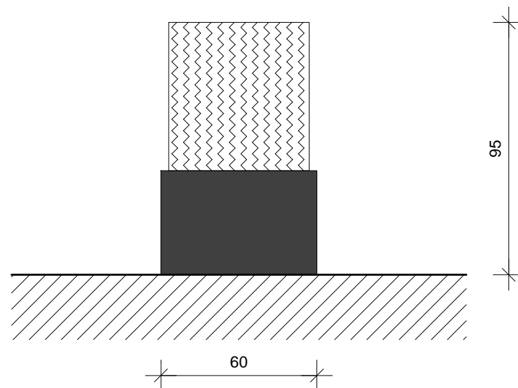
PRIJEDLOG 09 - TEGLE
