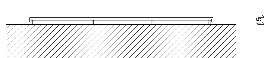
TLOCRT / POGLED PODIJA TERASE KOD PJEŠAČKIH ZONA NERAVNIH PLOHA
