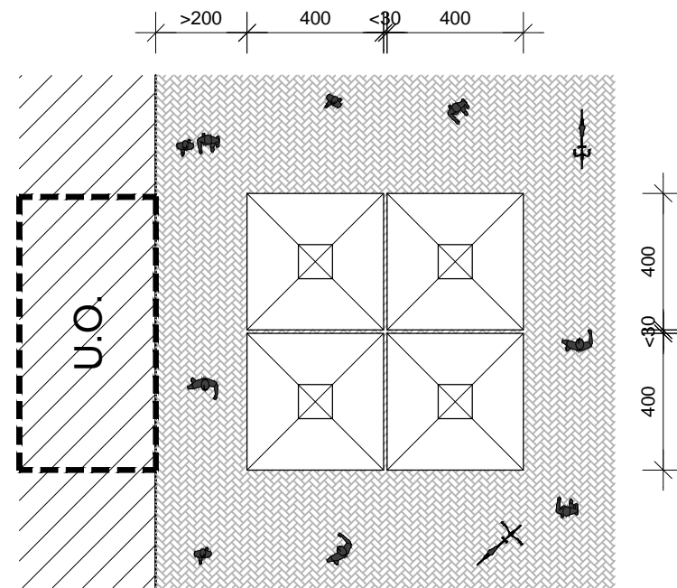
TLOCRT ČETIRI SOLITERNA SUNCOBRANA
