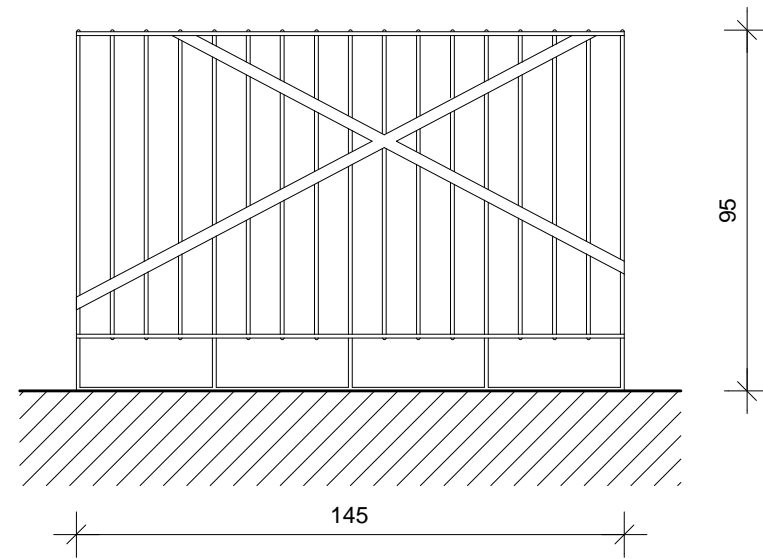
PRIJEDLOG 05 - ALUMINIJ
