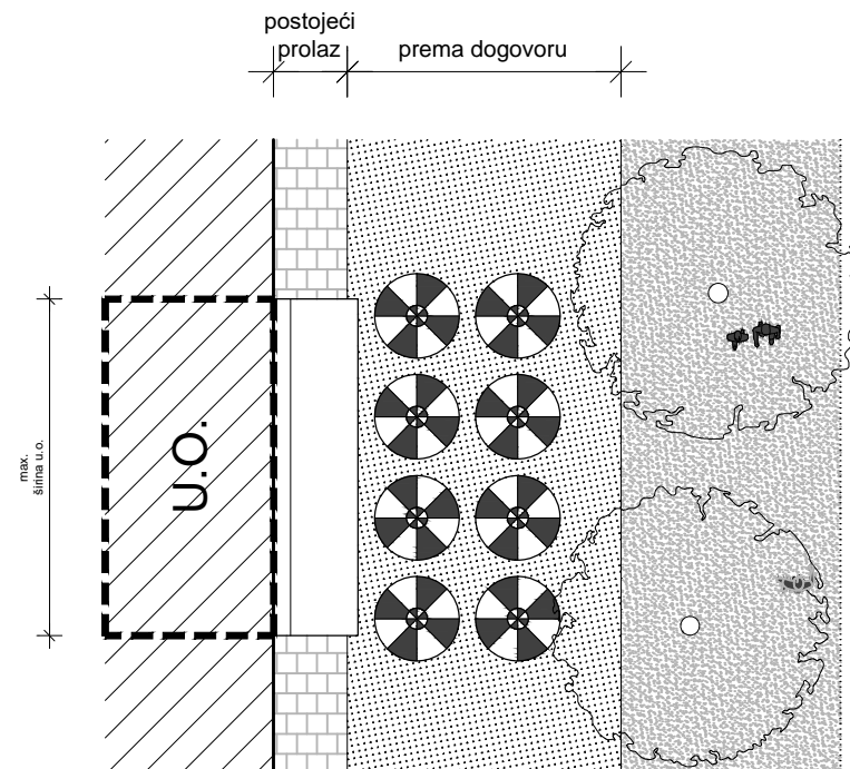
TLOCRT JEDNOSTREŠNIH TENDI U KOMBINACIJI SA SOLITERNIM MALIM SUNCOBRANIMA
