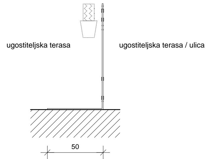
POGLED - PRIJEDLOG 01
