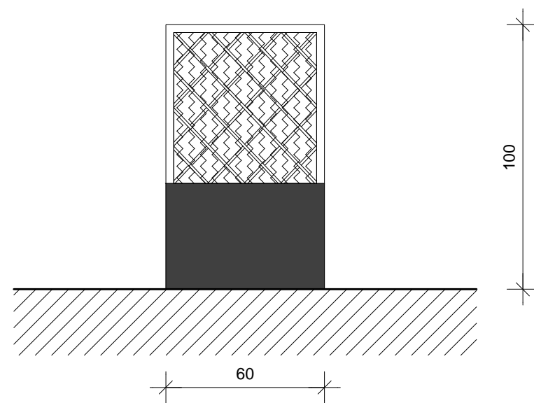
PRIJEDLOG 06 - TEGLE SA UGRAĐENIM RAŠLJAMA
