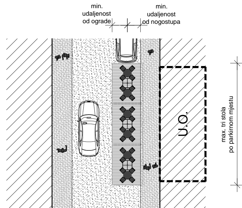
TLOCRT RASPOREDA NAMJEŠTAJA
