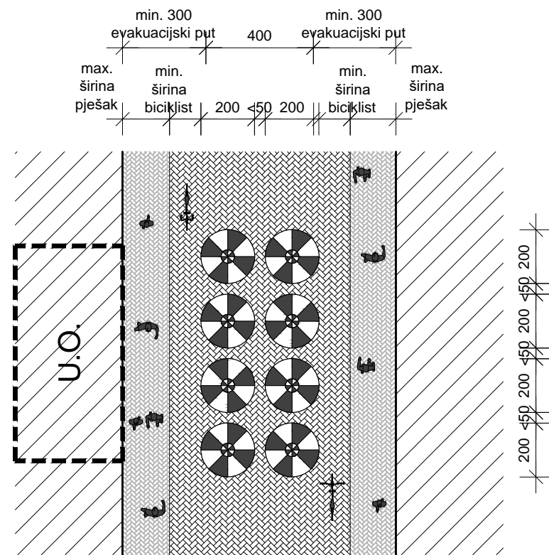
TLOCRT MALIH SOLITERNIH SUNCOBRANA
