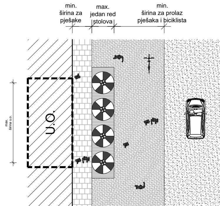
TLOCRT MALIH SOLITERNIH SUNCOBRANA
