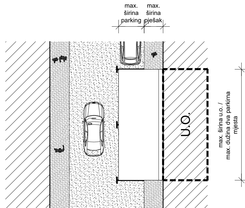
TLOCRT JEDNOSTREŠNE TENDE
