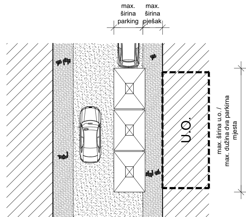
TLOCRT SREDNJIH SOLITERNIH SUNCOBRANA
