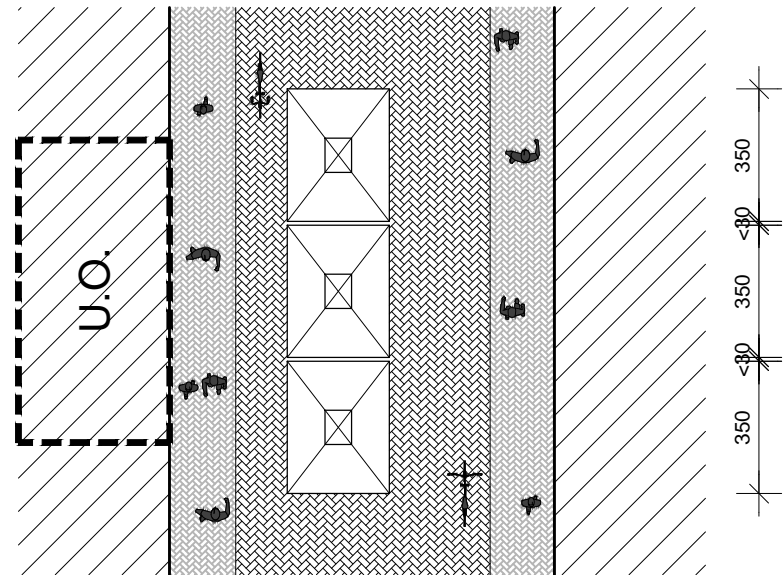
TLOCRT SREDNJIH SOLITERNIH SUNCOBRANA
