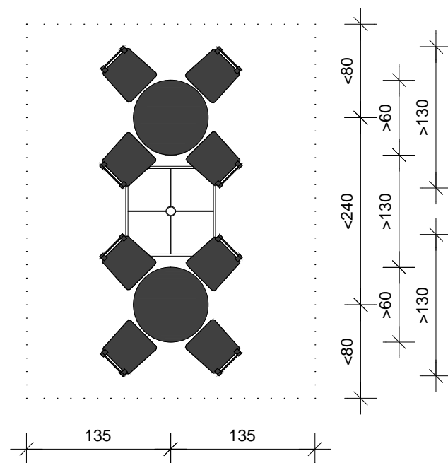
TLOCRT RASPOREDA NAMJEŠTAJA
