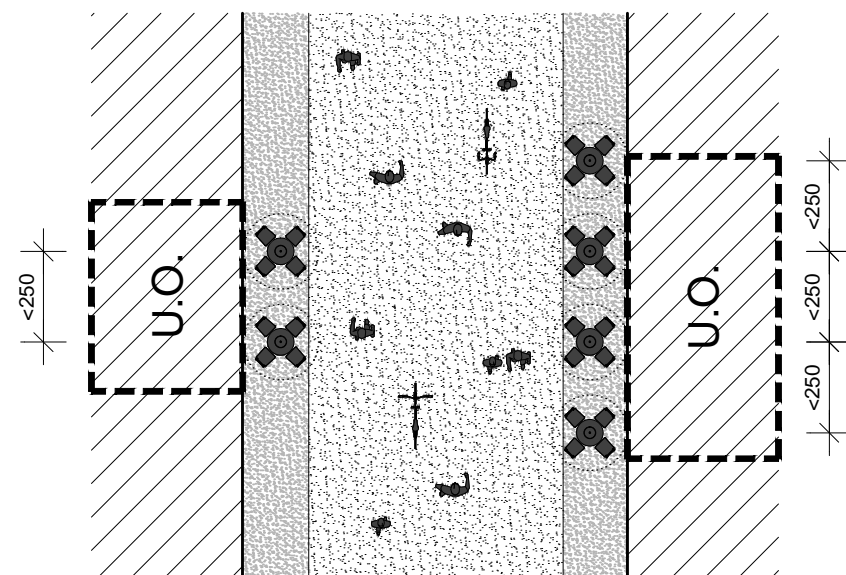
TLOCRT RASPOREDA NAMJEŠTAJA
